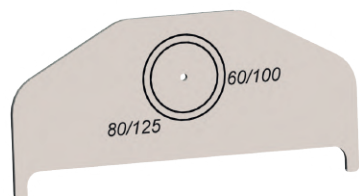
GABARIT DE PERÇAGE FLOVEA POUR FIXATION DE VENTOUSE
